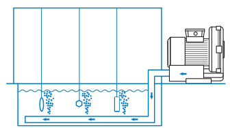
MIESZADŁA ELEKTROLITÓW W PRZEMYSŁE CHEMICZNYM
