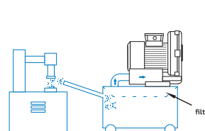
ODSYSANIE PYŁU PRZEMYSŁOWEGO
