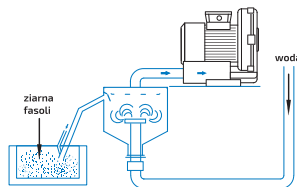
URZĄDZENIA DO MYCIA PRODUKTÓW SPOŻYWCZYCH
