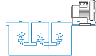
NAPOWIERZANIE OBSZARÓW HODOWLANYCH, FARM RYBNYCH
