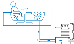
TWORZENIE BABELKÓW W WANNACH Z HYDROMASAŻEM
