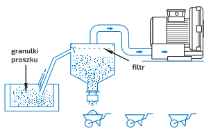
URZĄDZENIA DO TRANSPORTU GRANULEK PROSZKU
