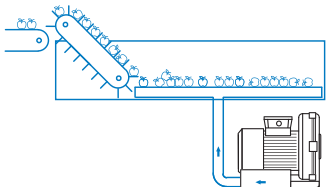
MYJKI WARZYW I OWOCÓW
