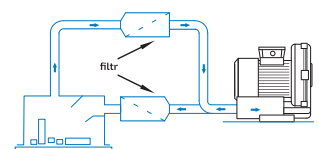
INSTALACJA USUWANIA PYŁU
