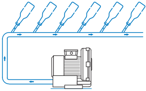
SUSZENIE BUTELEK
