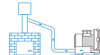
DOPROWADZENIE POWIETRZA DO PIECÓW
