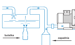
MASZYNY DO NAPEŁNIANIA BUTELEK
