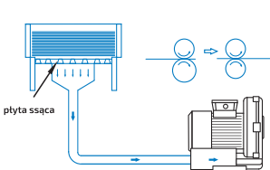
TRANSPORT PAPIERU, TEKSTURY
