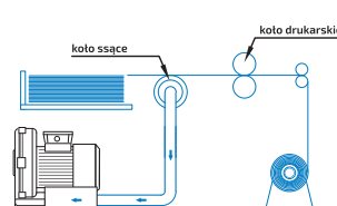
PRZENOŚNIK PAPIERU W DRUKARNIACH
