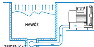
FERMENTACJA
