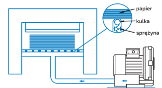
PODTRZYMANIE BLOKU PAPIERU W PROCESACH CIĘCIA
